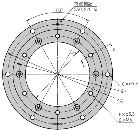
[安裝孔加工圖]
