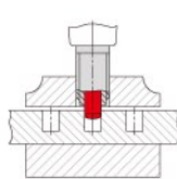
夾持力解除後仍然保持定位
