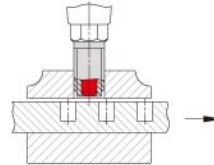
夾持力解除且定位移除後，工件始可以移動
