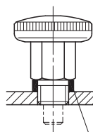
調整環 SGR609.5
