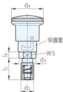
圖1 銷子內藏
