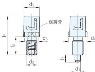
圖2 銷子內藏 銷子外伸鎖固
