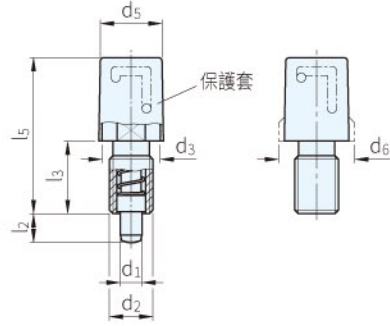
圖2 銷子外伸
