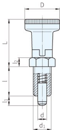
圖1(無螺帽)
