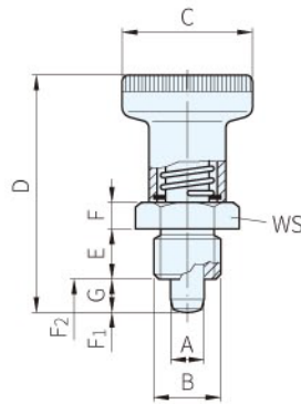
圖1(無卡鎖)
