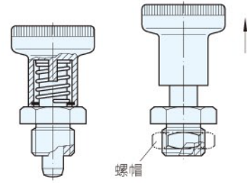
圖2(有卡鎖)
