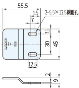
吸片 GS-AS-YN005F (平面安裝規格)
