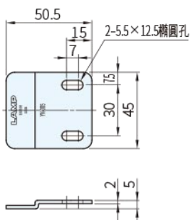
吸片 GS-AS-YN005D (落差安裝規格)
